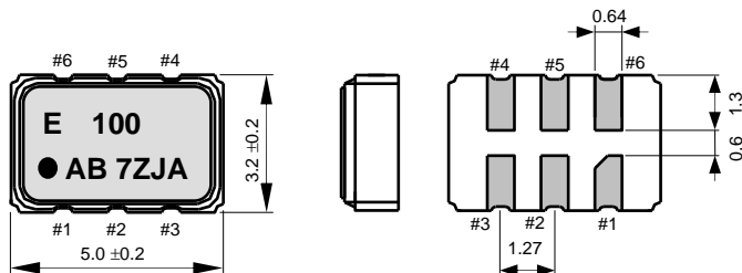
引脚图
